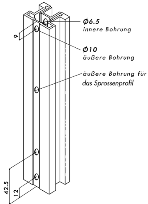
Bohrbild Senkrechtprofil
