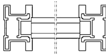
Querschnitt Schiebetürflügel
